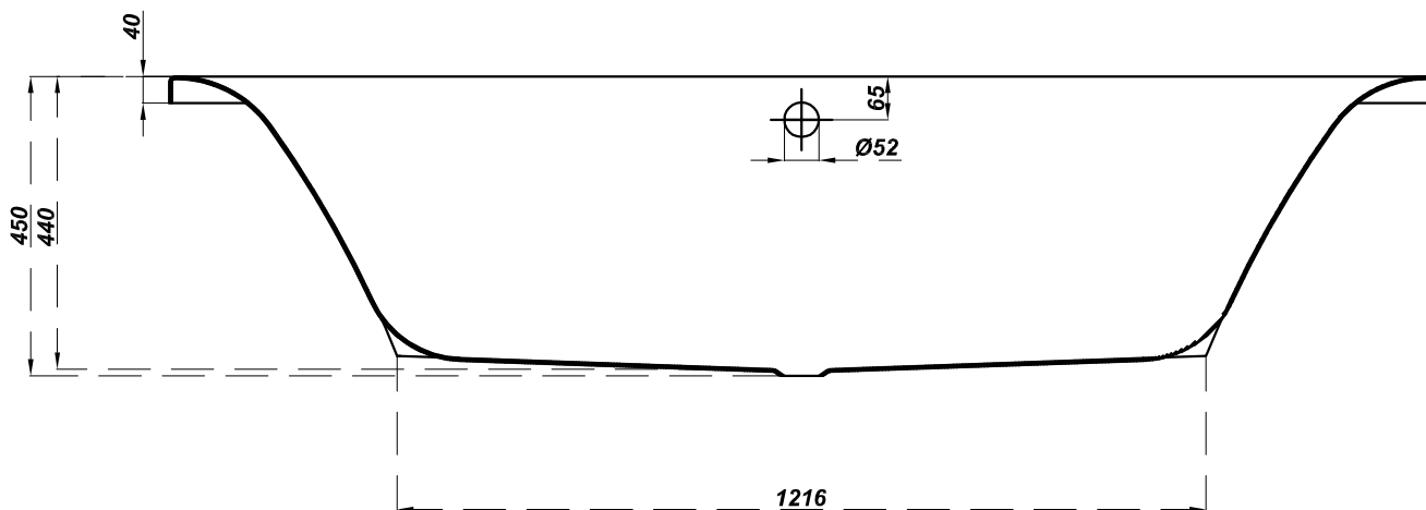
A-A ( 1 : 8 )
